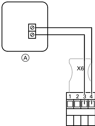
(A) Außentempersensor
