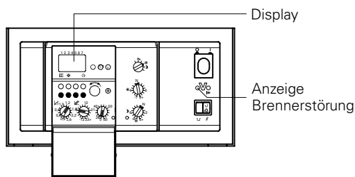
Regelung für witterungsgeführten Betrieb mit Standard-Bedieneinheit
