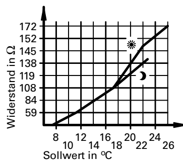
Fernbedienungsgerät-RS
